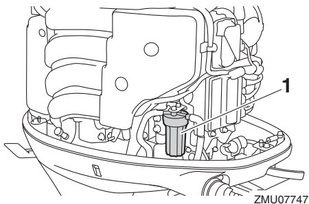
1. Kraftstofffilter
