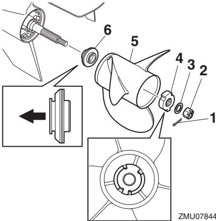
1. Sicherungssplint
