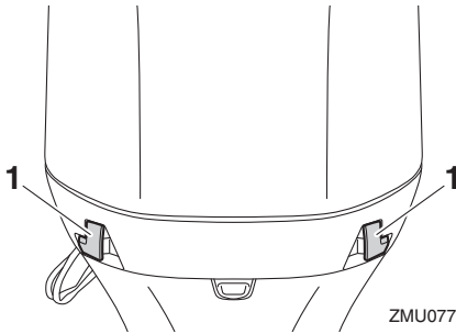
1. Levier de verrouillage du capot
