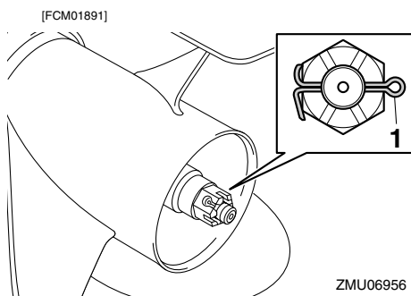
1. Goupille fendue
