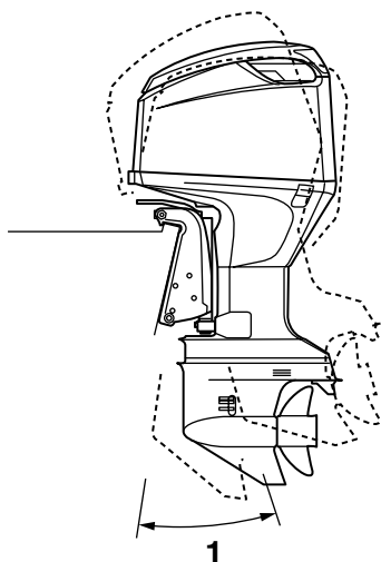
1. Trimm-Betriebswinkel
