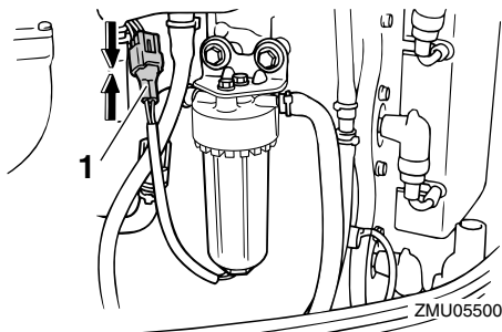
1. Wasseranzeigeschalter-Stecker
