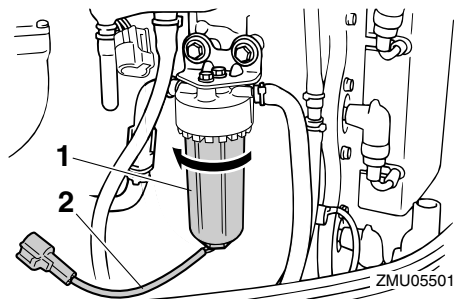
1. Filtergehäuse 2. Wasseranzeigeschalter-Kabel
