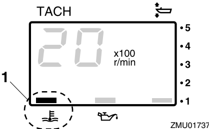
1. Überhitzungs-Warnanzeige
