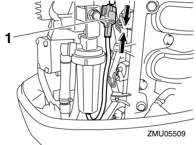
1. Wasseranzeigeschalter-Stecker
