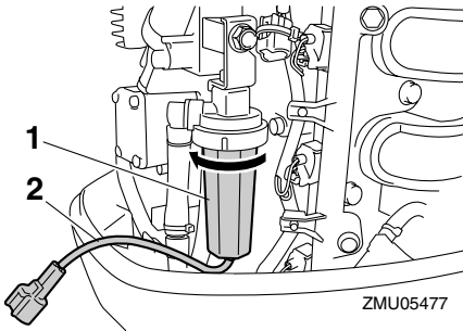
1. Filtergehäuse 2. Wasseranzeigeschalter-Kabel
