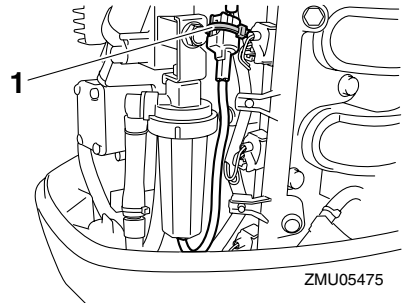
1. Kabelbinder
