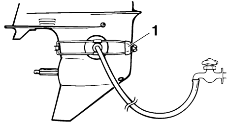
1. Spülaufsatz
