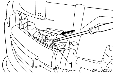
1. Chokekoppelstang
