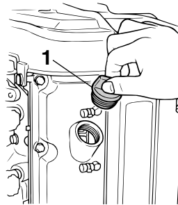
1. Bouchon de remplissage d'huile
