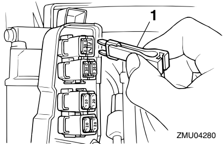
1. Zekeringtrekker
