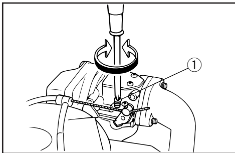
① Tomgangsskrue
