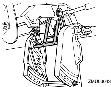
1. Motorhauben-Verriegelungshebel
