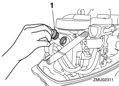
1. Oljepåfyllningskåpa
