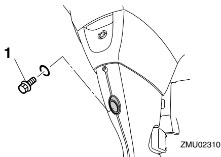
1. Dräneringsskruv
