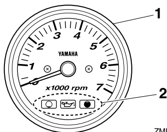
1. Drehzahlmesser
