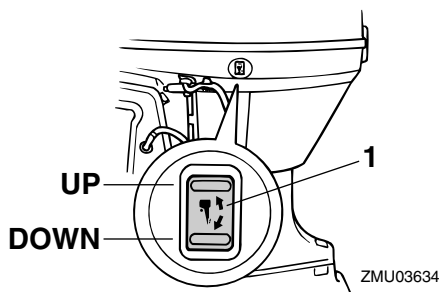
1. PTT-Schalter
