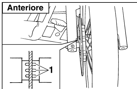
1. Scanalatura indicatore d'usura pastiglia freno (x 3)
