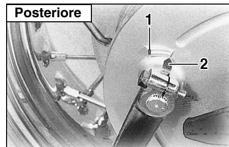
1. Linea del limite di usura ganasce freno 2. Indicatore di usura ganasce freno
