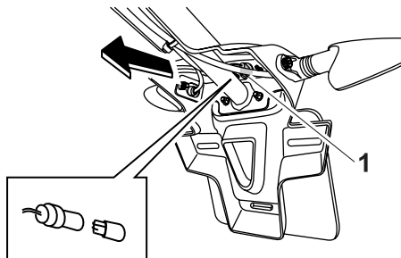
1. Lampada luce targa
