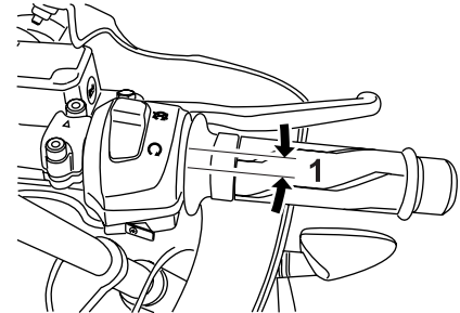
1. Gioco del cavo dell'acceleratore
