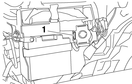
1. Reservezekering
