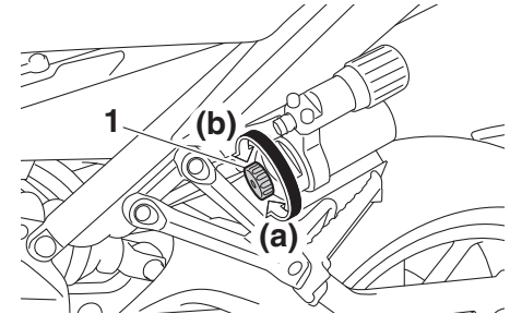
1. Druckstufendämpfungs-Einstellknopf
