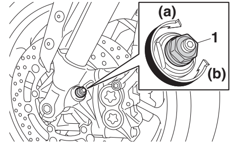
1. Druckstufendämpfungs-Einstellschraube (für schnelle Dämpfung)
