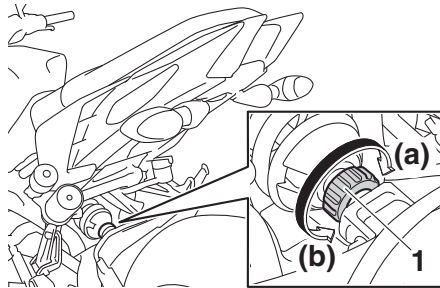
1. Zugstufendämpfungs-Einstellknopf
