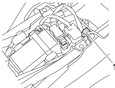
1. Diagnose-Steckverbinder
