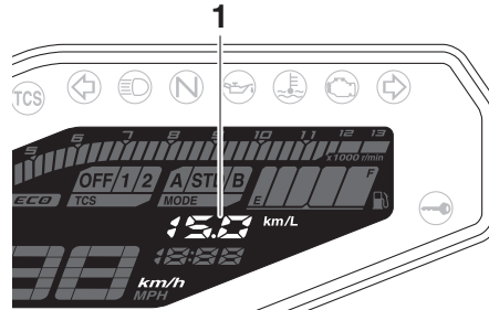
1. Momentane Kraftstoffverbrauchsanzeige
