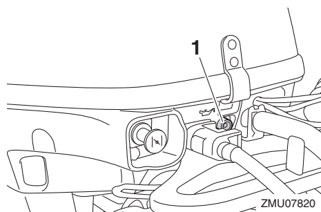
1. Oliegedrukschuwingslampje
