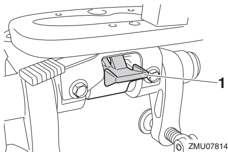
1. Kantelvergrendelhendel
