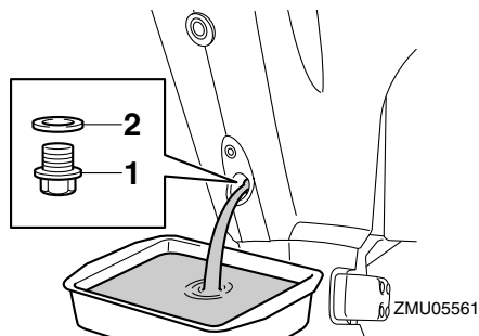
1. Aftapschroef 2. Pakking
