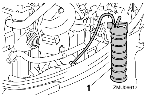
1. Olieververser
